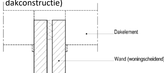
Verticale doorsnede
